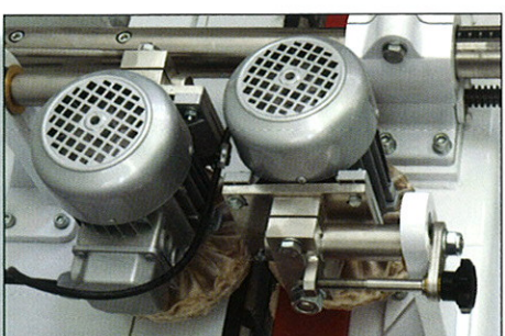
PC-2 BUFFING UNIT GRUPO PULCANTOS GRUPPO SPAZZOLE 0,05 + 0,05 kW / 1500 RPM, Ø 100 mm COTTON DISCS DISCOS DE ALGODÓN DISCHI DI COTONE (OPTIONAL OPCIONAL OPZIONALE)
