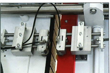
RR-8 GLUE SCRAPER UNIT GRUPO RASCADOR DE PEGAMENTO GRUPPO RASCHIACOLLA FLOATING BLADES CUCILLAS FLOTANTES UTENSILI FLUTANTI AIR BLOWERS SOPLADORES AIRE UGELLI DE SOFIAGGIO (OPTIONAL / OPCIONAL / OPZIONALE)
