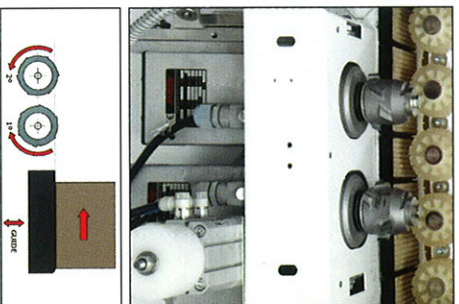
PF-2 PRE MILLING UNIT TUPI DE ENTRADA GRUPPO RETTIFICHE (FLEXY P/FLEXY PC) 1,1 + 0,75 kW / 12000 RPM PNEUM. THRUST / PRESIÓN NEUM. PRESS. PNEUM. DIA 100S / HTAS / FRESE H30 (STD.) H55 (OPT.)
